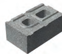
Leca® Block 300 Hörn
