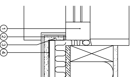
DETALJ 1 Skala 1:5
